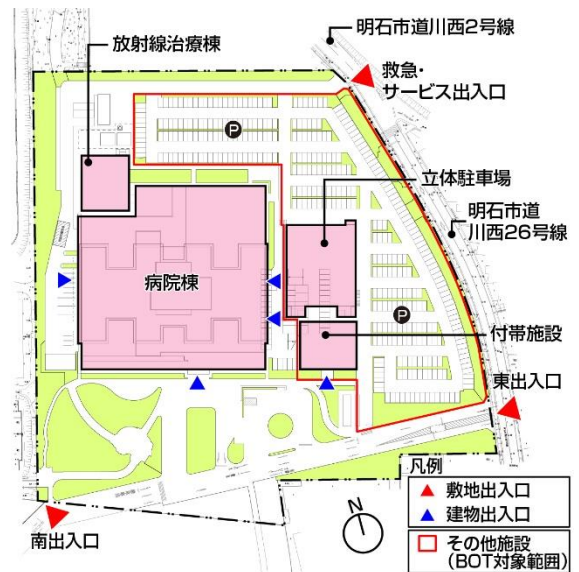
敷地平面図
